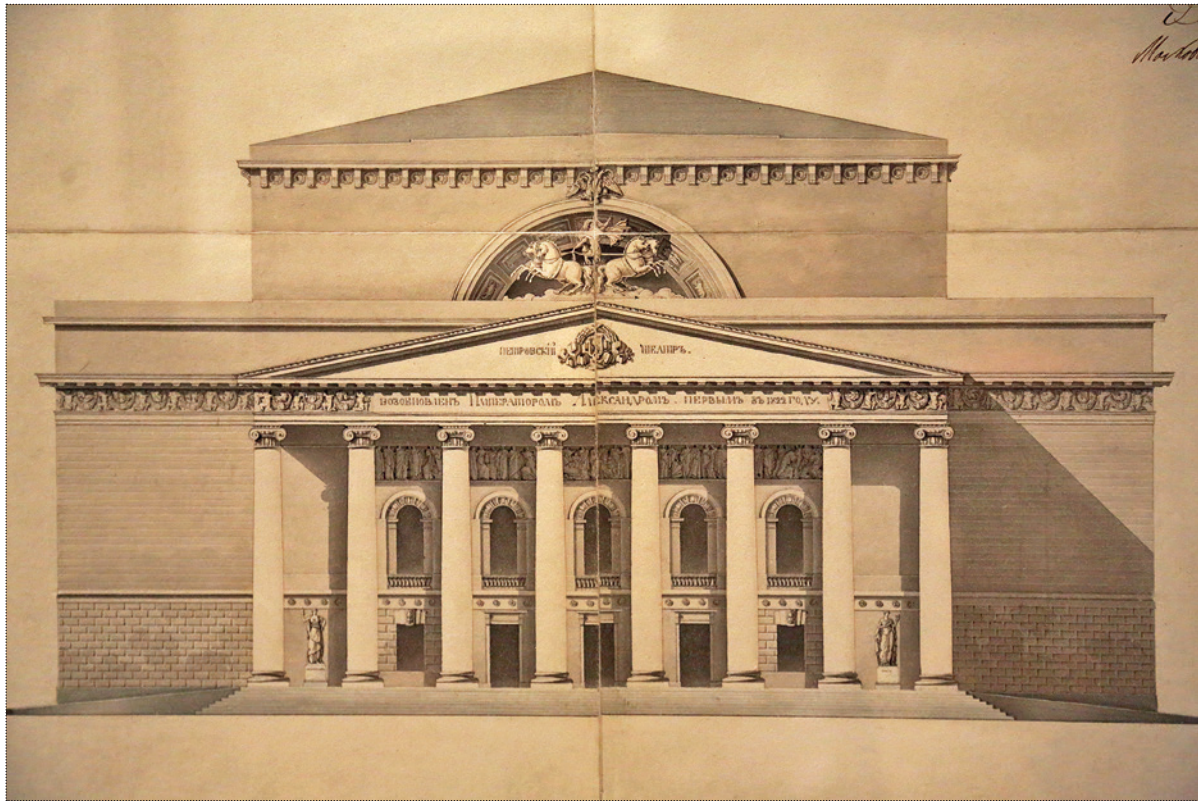
Проект Большого Петровского театра в Москве. Главный фасад. Фрагмент. О. Бове. 1821 год
