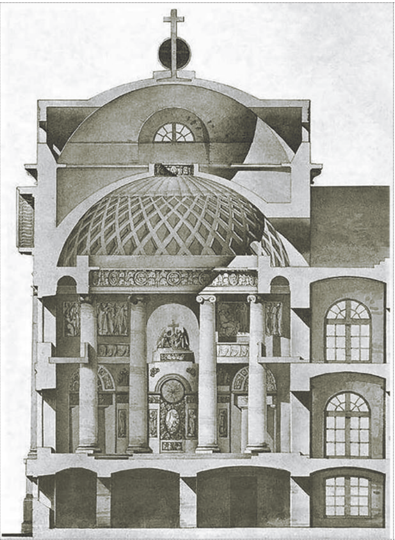
Первая Градская больница. Церковь-ротонда. Поперечный разрез. Проект О.И. Бове. 1827 год. РГИА
