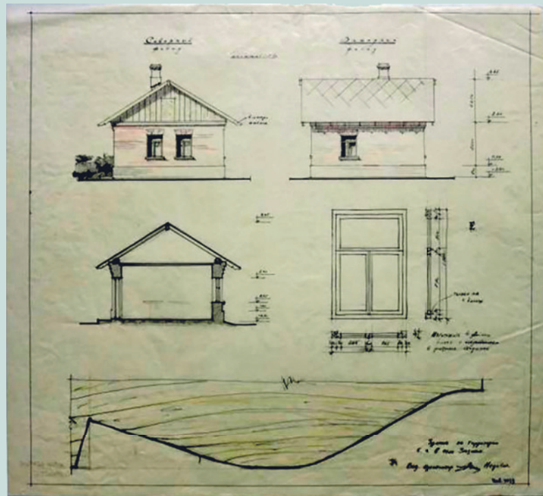
Обмерный чертёж хозяйственной постройки у церкви Бориса и Глеба в Зюзине. Н.Д. Недович. 1960-е годы. ГНИМА им. А.В. Щусева
