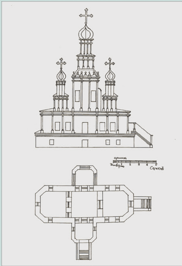
Фасад и план церкви Бориса и Глеба села Зюзина, приложенный к рапорту Пехрянской десятины благочинного священника Романа Стефанова, пославшего запрошенные Синодом документы 13 апреля 1788 года
