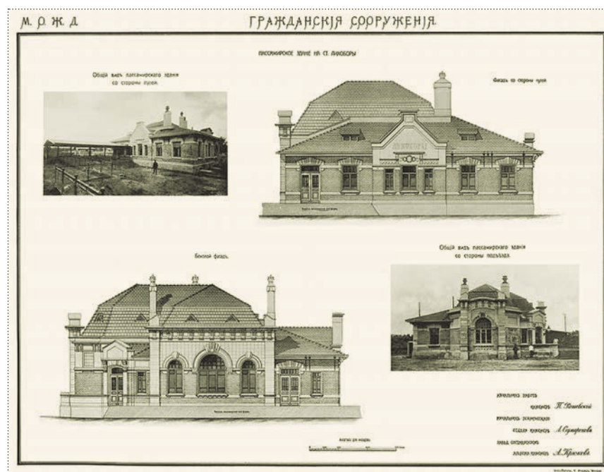
План пассажирской станции Лихоборы. «Альбом исполнительных чертежей 1903–1908 года»
