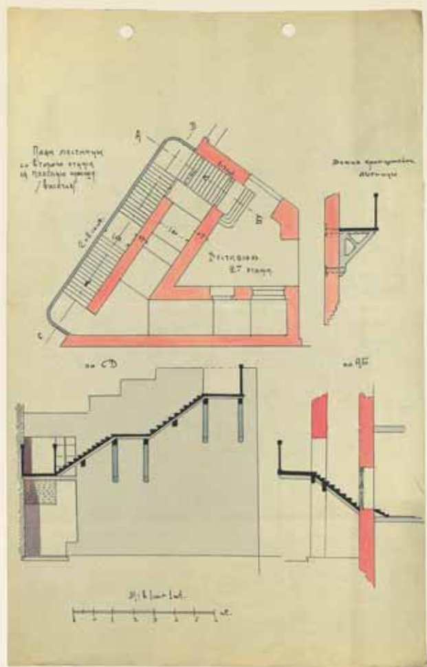
Проект устройства лестницы на крышу в здании конторы Ново-Сухаревского рынка. 1925 г. ЦГА Москвы. Ф. Р-1275, оп. 1, д. 197, л. 3
